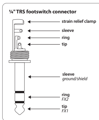
Fig. 4.4: Conector de jack mono para pedal
